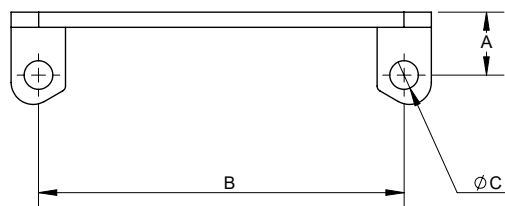
B5107-Series Bracket - 8"
