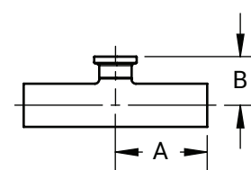
BPE Table DT-4.1.2-7 ASME BPE 2019
