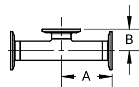
BPE Table DT-4.1.2-5 ASME BPE 2019
